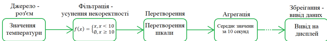
Рисунок 1. Приклад опрацювання даних в потоках.
