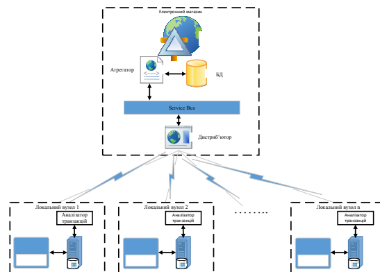
Рисунок 1. Архітектура розподіленої комп'ютерної системи збору та управління даними електронної комерції
