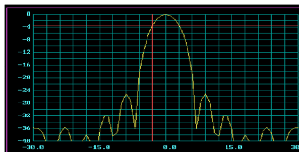
Рисунок 3. ДС антени.
