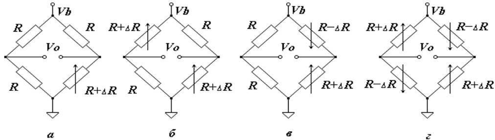
Рисунок 1. Конфігурації включення тензодавачів в мостові схеми.
