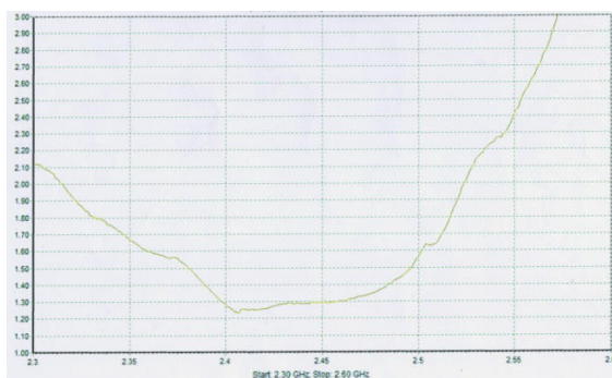
Рисунок 2. VCWR антени.
