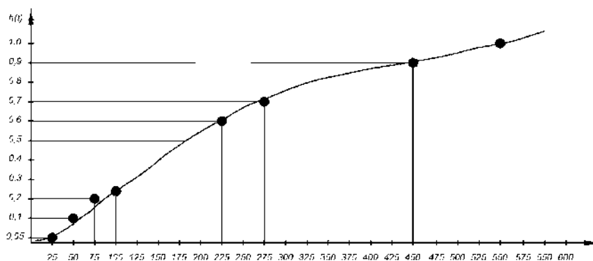
Рисунок 2. Графік кривої розгону перехідної функції Wp(p)
