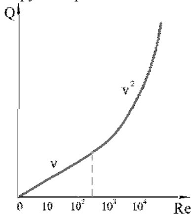
Рисунок 1. Залежність сили лобового опору від числа Рейнольдса
